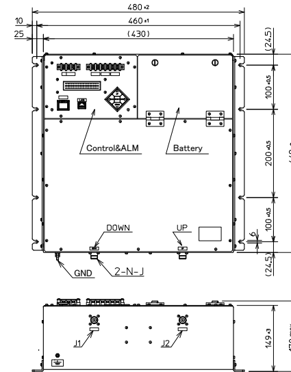
外観図
