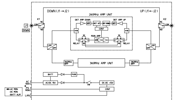
ブロック図
