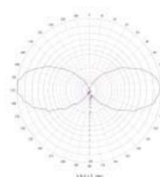
垂直面㉑
