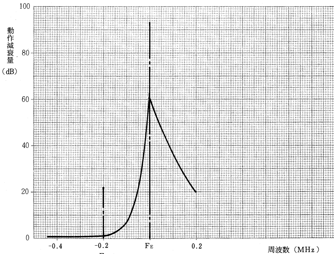
減衰特性例
