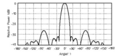
指向性特性例
