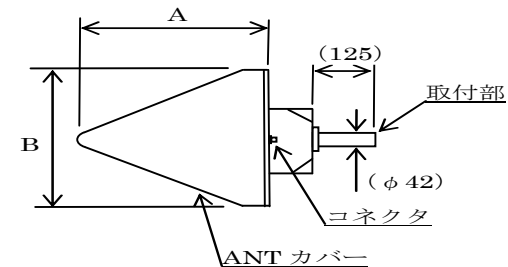
LP-06301R 外観図
