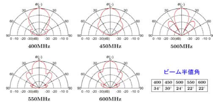
垂直面(YZ面) E_{\phi} 成分 放射パターン
